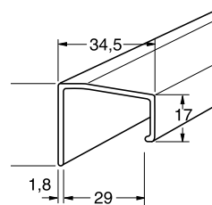
Ukončovací profil B
