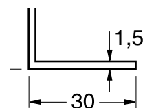
Krycí rohová lišta 30/20
